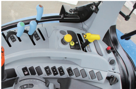
右横コンソールにまとめられた作業操作装置
